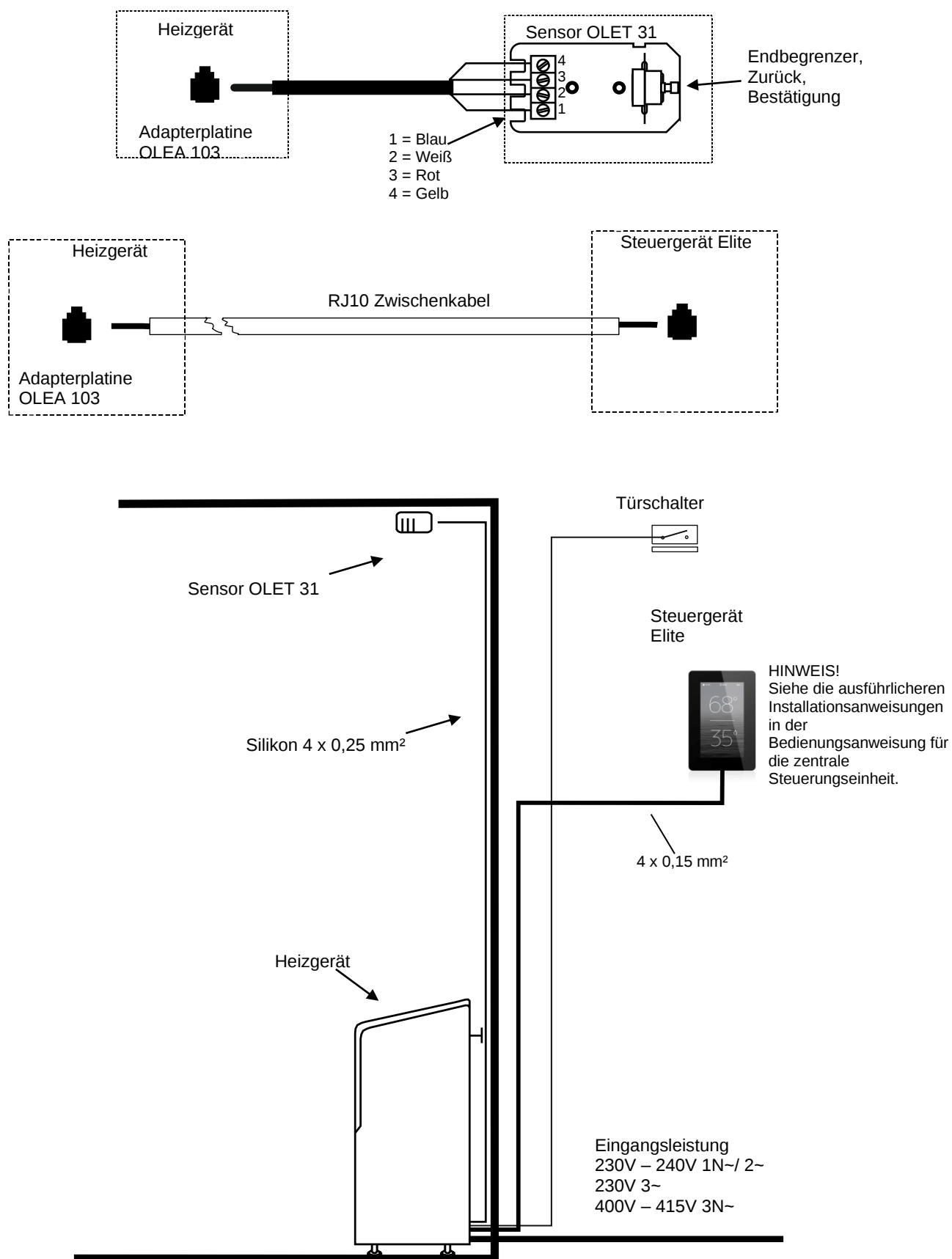
Abbildung 9 Prinzipbild
