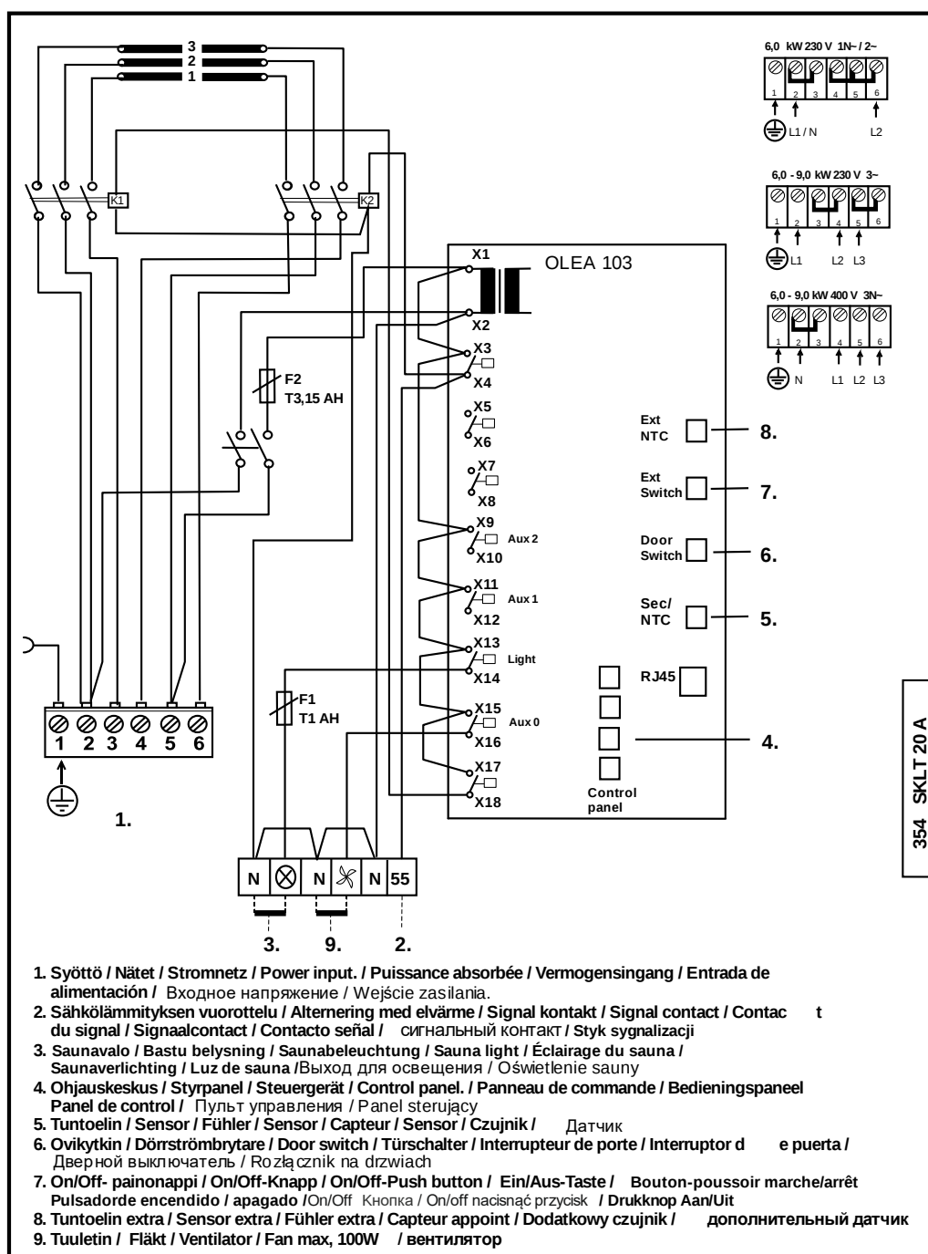
Imagen 6. Diagrama de conexiones
