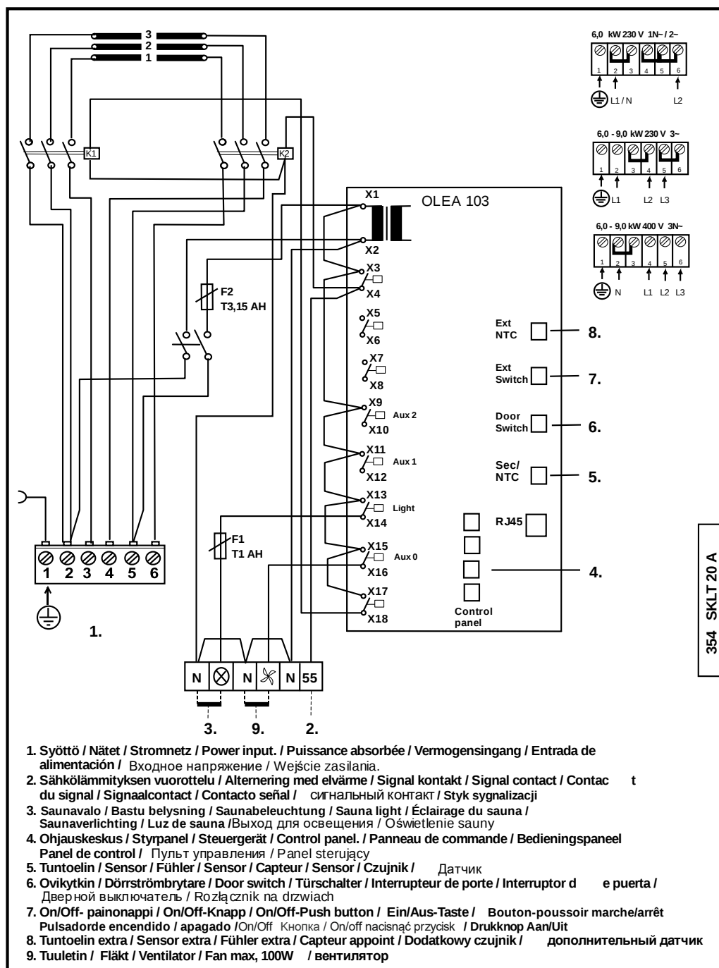
Kuva 6. Kytkentäkaava
