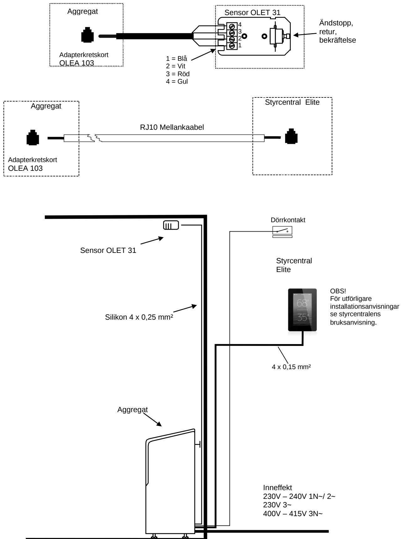
Bild 9 Principskiss
