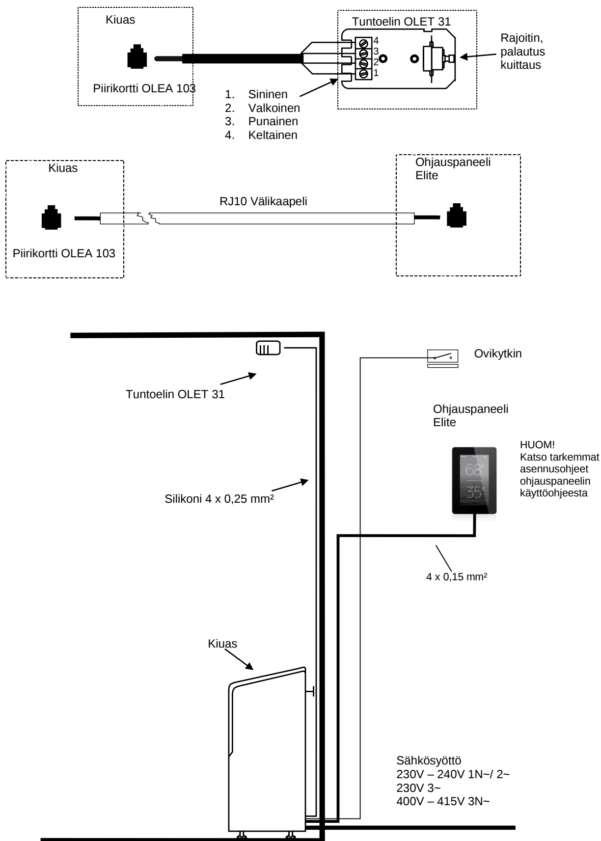
Kuva 9 Periaatekuva asennuksesta
