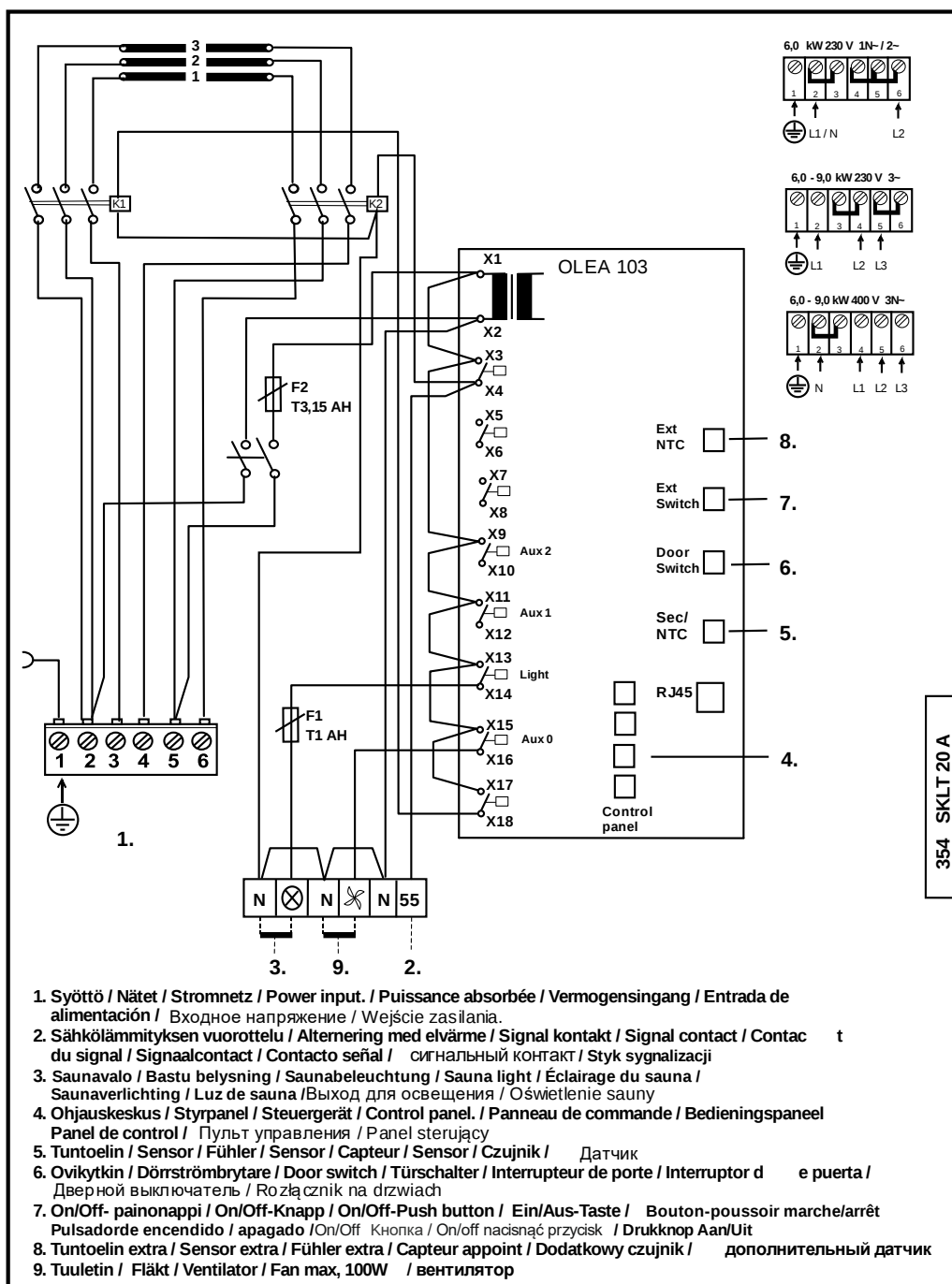
Bild 6. Kopplingsschema
