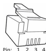
Stiftlayout på en RJ10-kontakt
