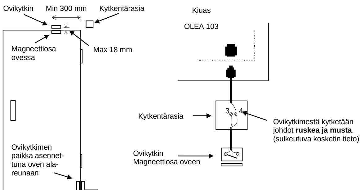
Kuva 7 Ovikytin asento
